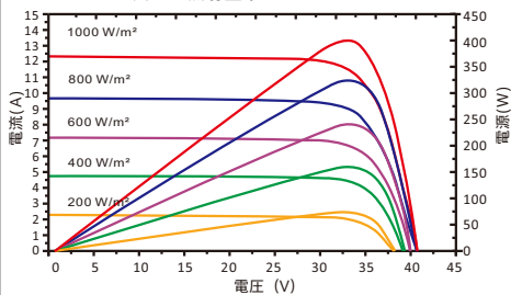
異なる照射量下での I-V カーブ
