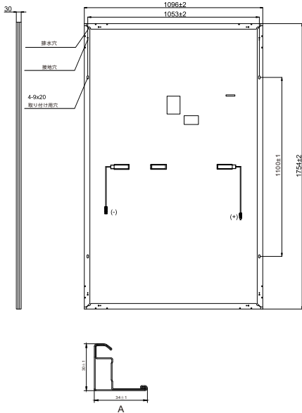
太陽光発電モジュール図面 単位: mm
