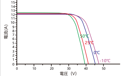
異なる温度下での I-V カーブ
